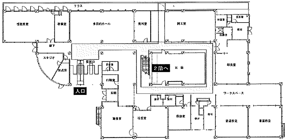
1階 平面図
