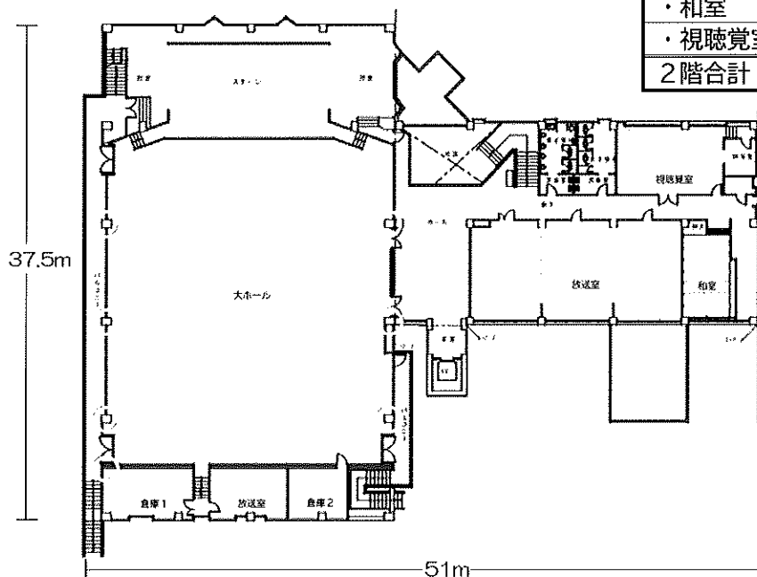
[2階]
