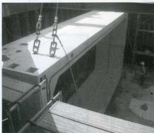
高浦橋の復旧工事 (ボックスカルバートを設置しています)
