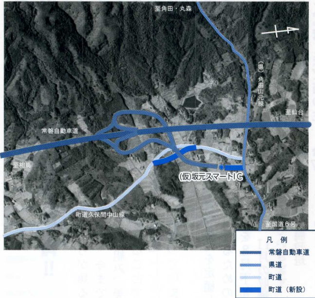
坂元スマートICイメージ図
