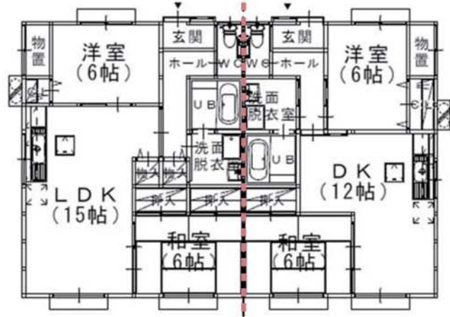
2LDK平屋平面図 3LDK1階 平面図
